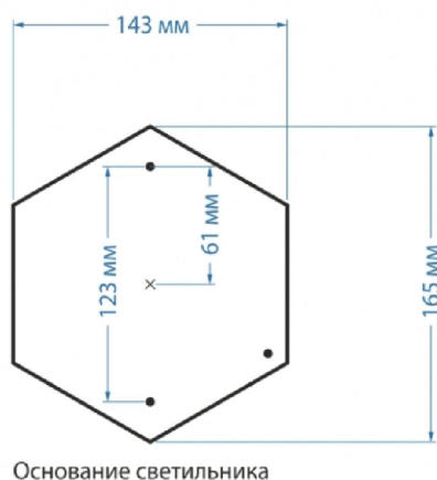
Основание светильника
